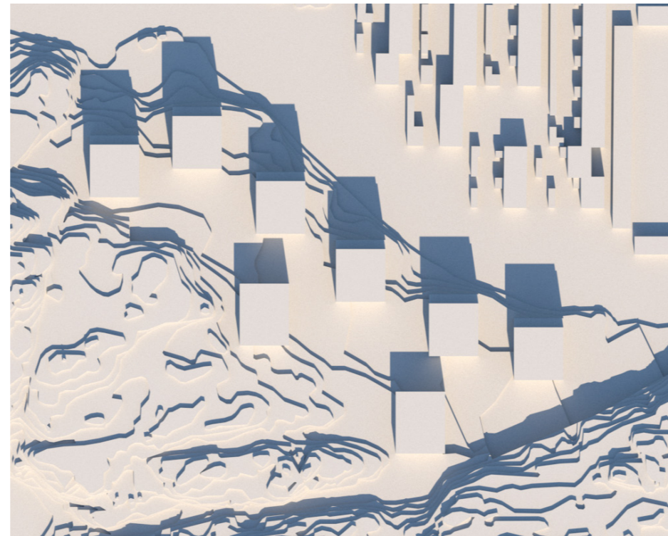
Vår-/höstdagjämning kl 12
