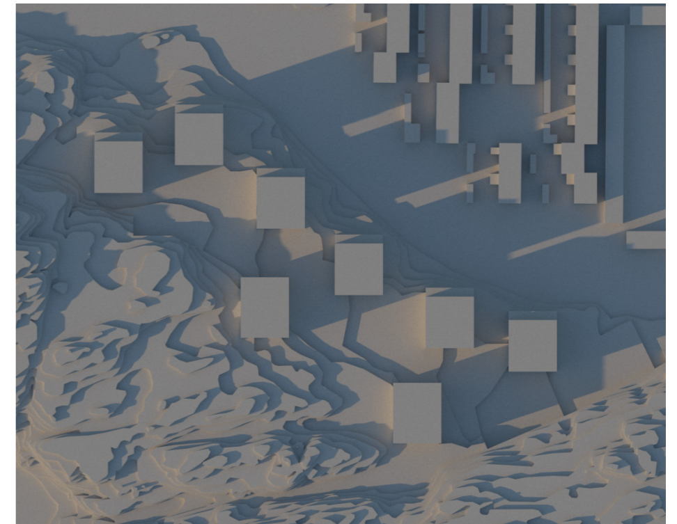
Vår-/höstdagjämning kl 18
