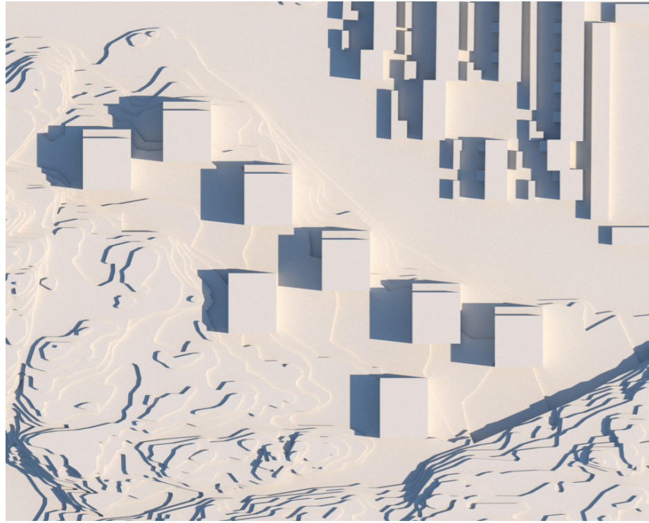
Midsommar kl 8
