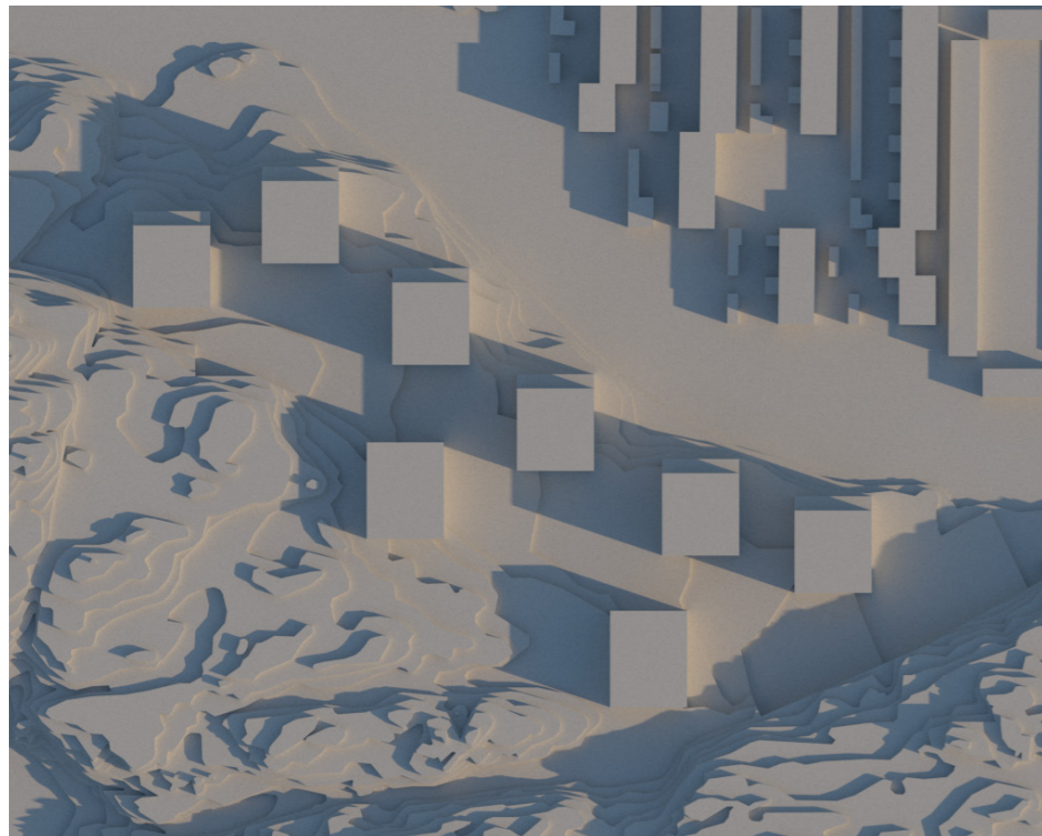
Vår-/höstdagjämning kl 8
